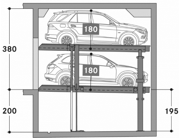
Figure 6 : schéma en coupe d'un système « park-lift »
