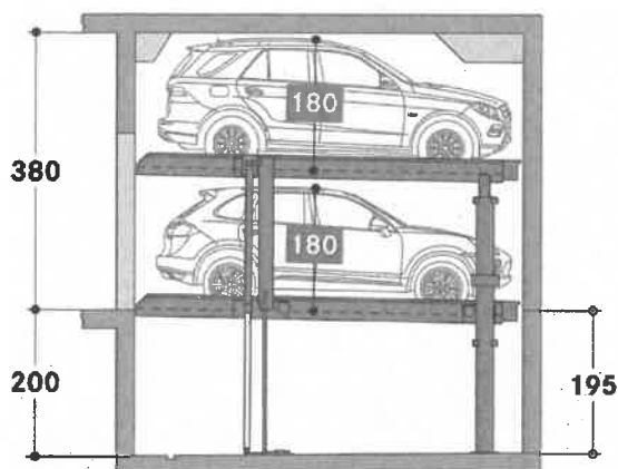
Figure 6 : schéma en coupe d'un système « park-lift »
